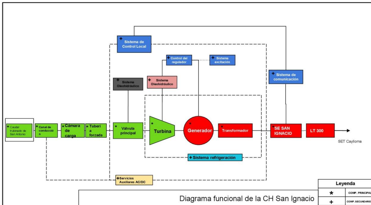
Figura N° 1. Diagrama de flujo de la CH San Ignacio
